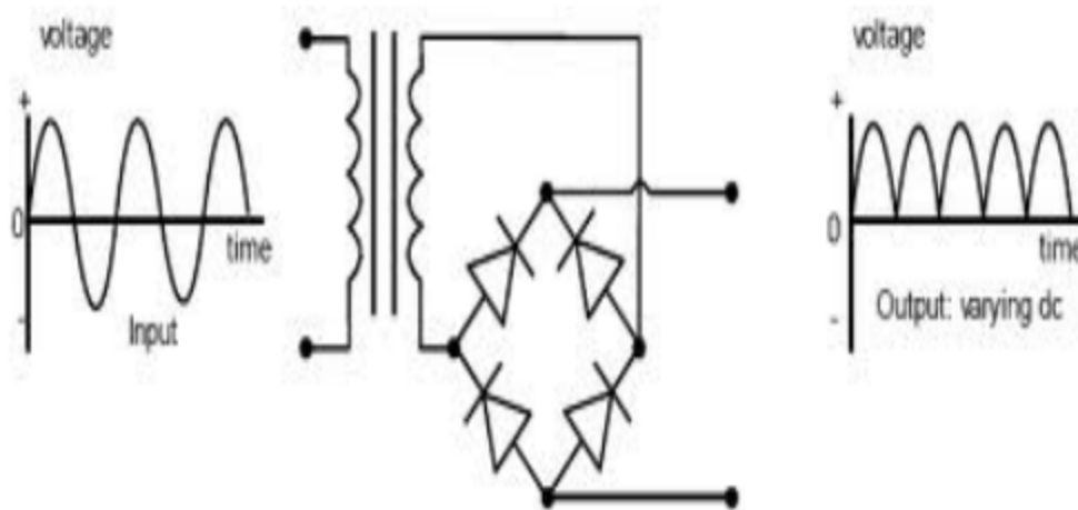
Figure : Rectifier
